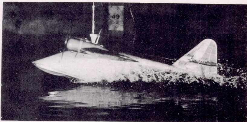
(b) C_V = 5.54 ; \tau = 11^\circ ; \delta_e = -10^\circ .
