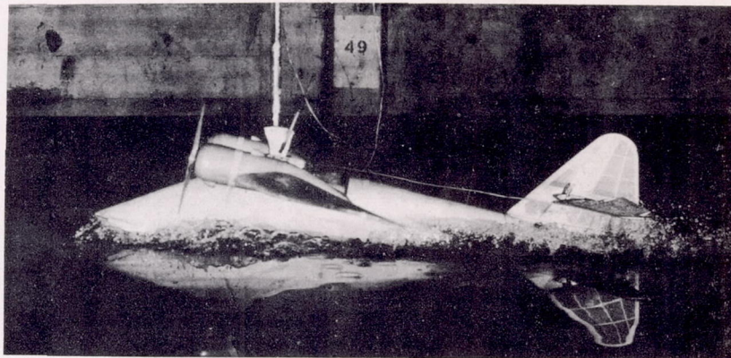
(a) C_V = 2.77 ; \tau = 9.8^\circ ; \delta_e = -15^\circ .
