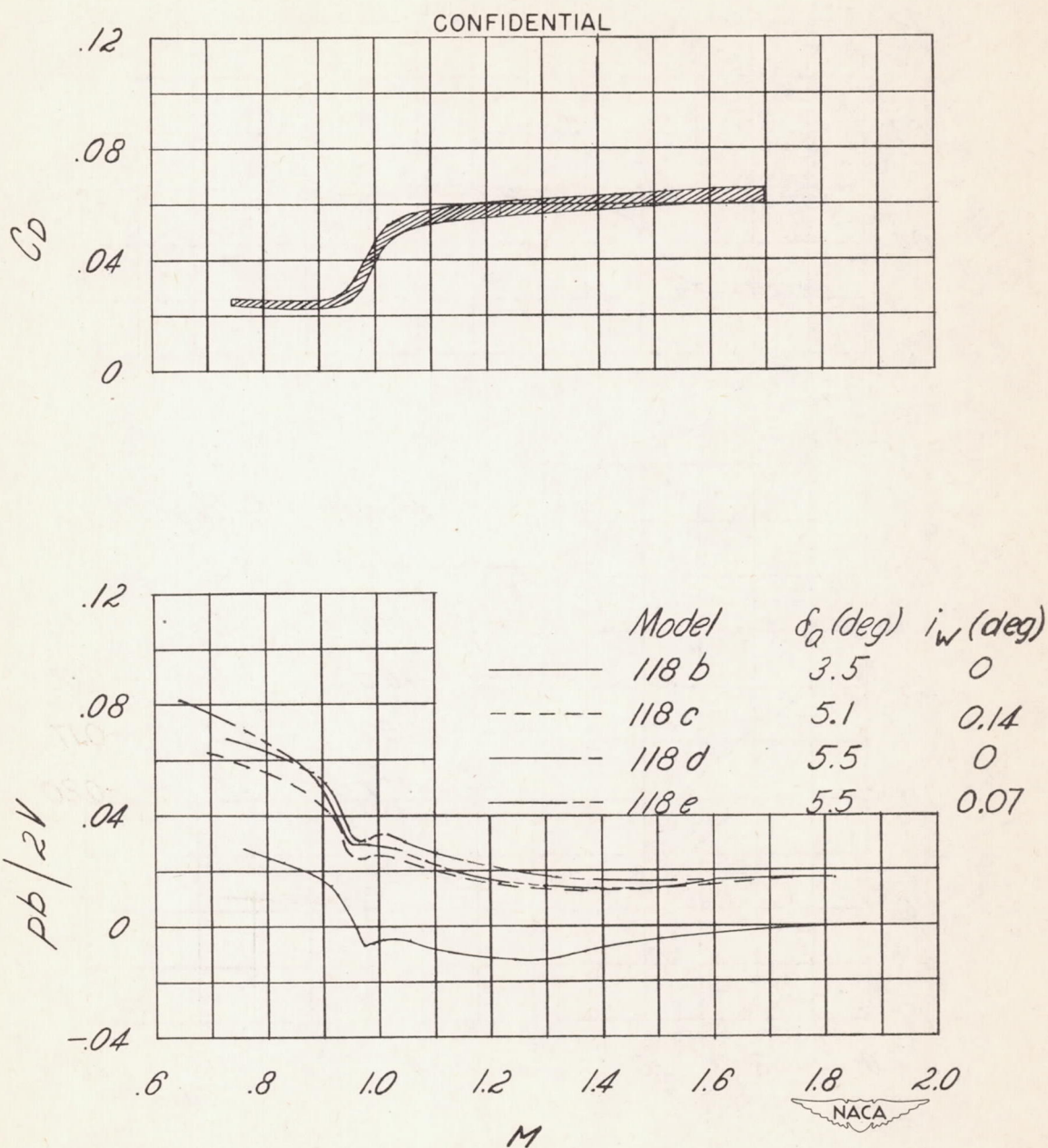
(d) 9-percent-thick circular-arc airfoil section.
