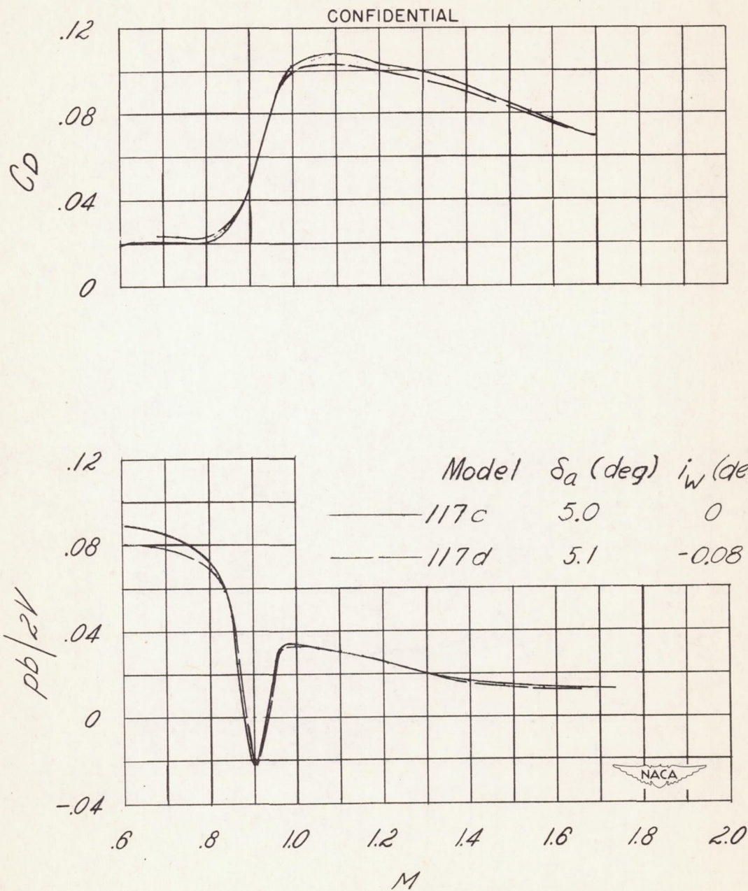
(d) 9-percent-thick circular-arc airfoil section
