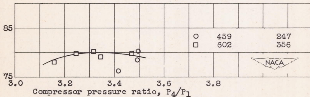
(d) Average compressor-inlet Reynolds number, 61,100.
