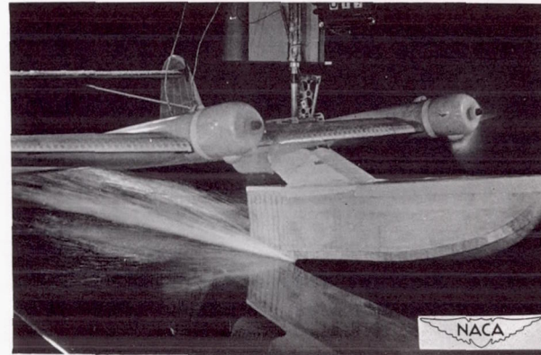
(d) C_V = 8.35 ; trim = 7.1^\circ .
