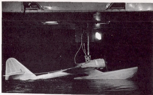
(a) C_V = 0 ; trim = 10.2°.
