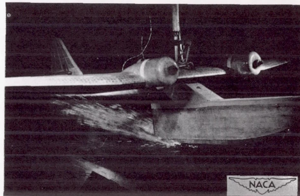
(d) C_V = 8.35 ; trim = 2.9°; (porpoising).
