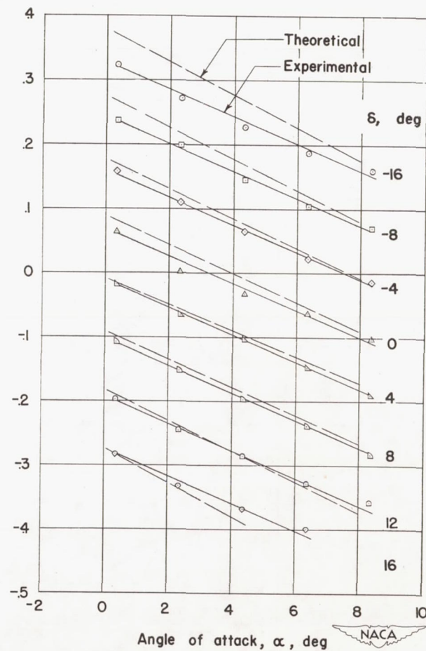
Fixed transition [configuration (d) Fig. 5]
