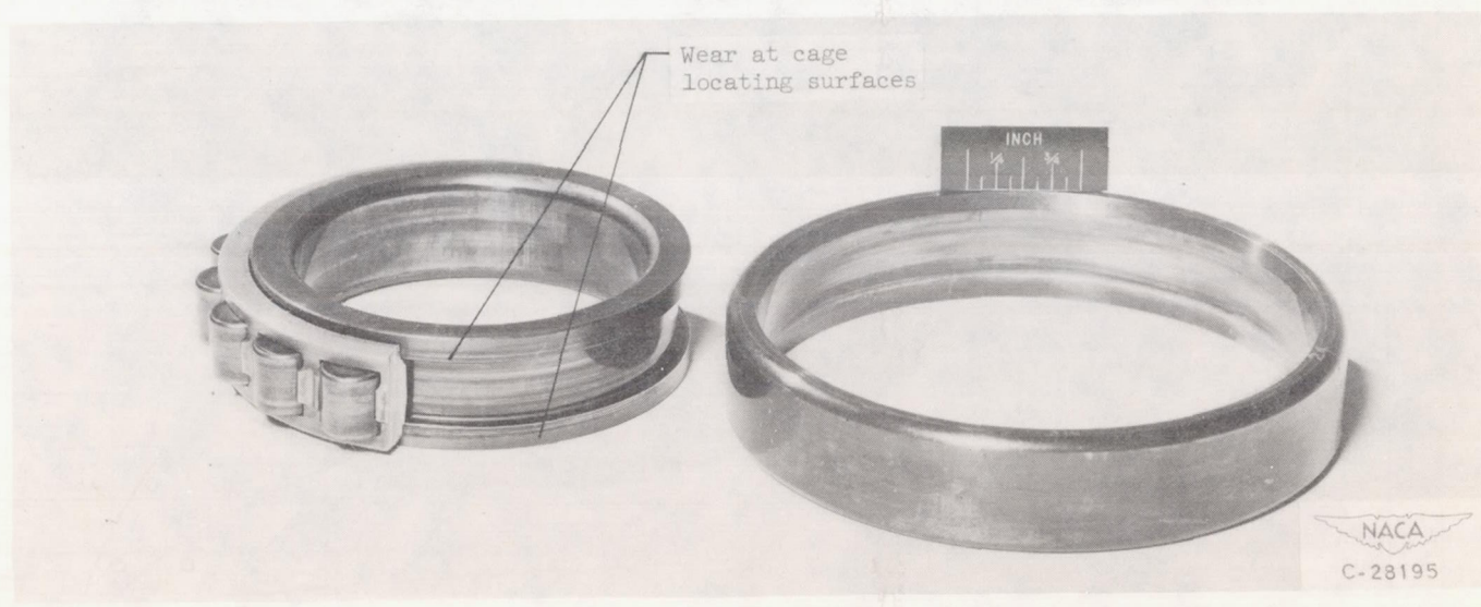
(d) Bearing 16.
