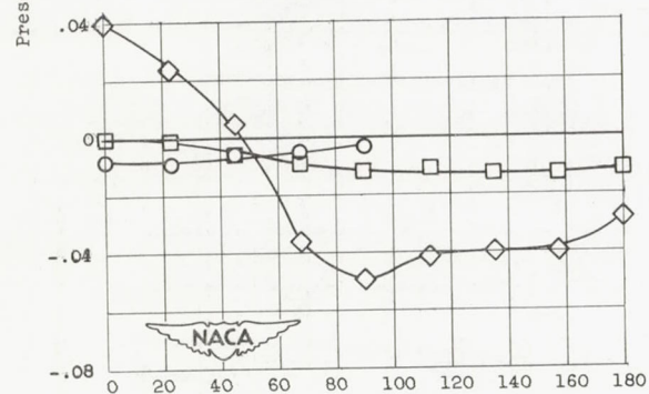
(d) Axial station, 1.291 feet; Reynolds number, 2 \times 10^6 .
