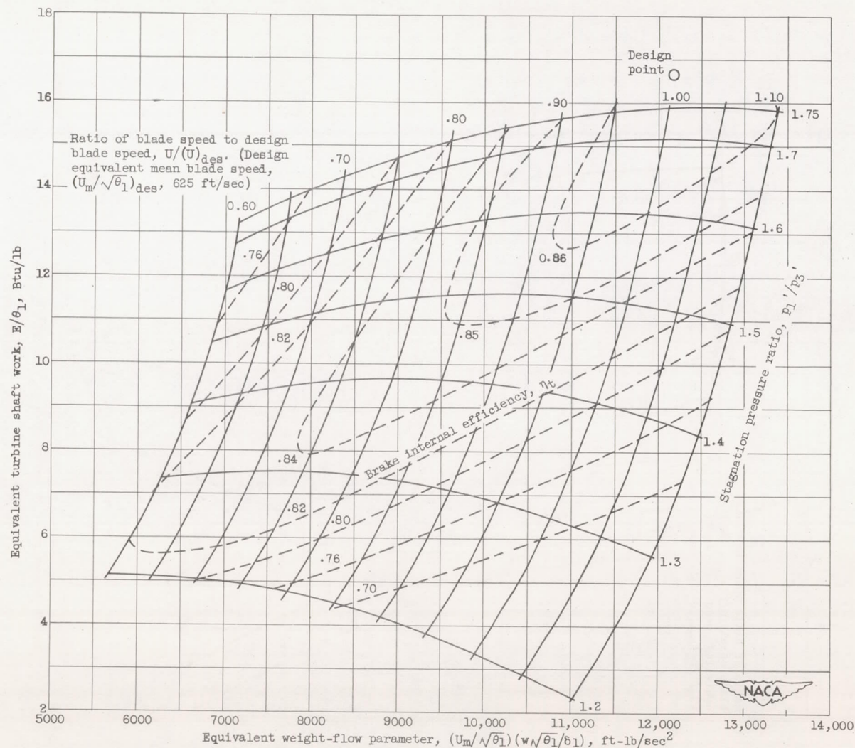
(d) 24-blade-rotor-turbine configuration.
