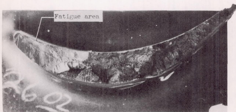
(b) Fatigue fracture.
