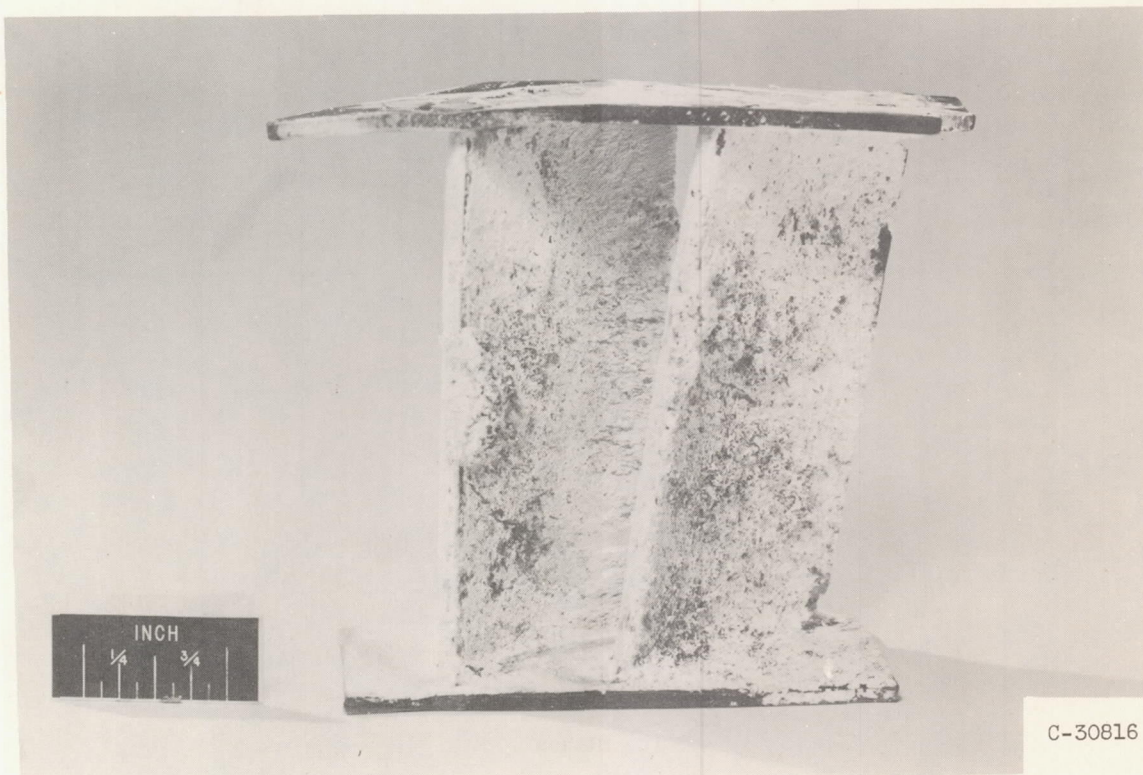
(b) Blades.
