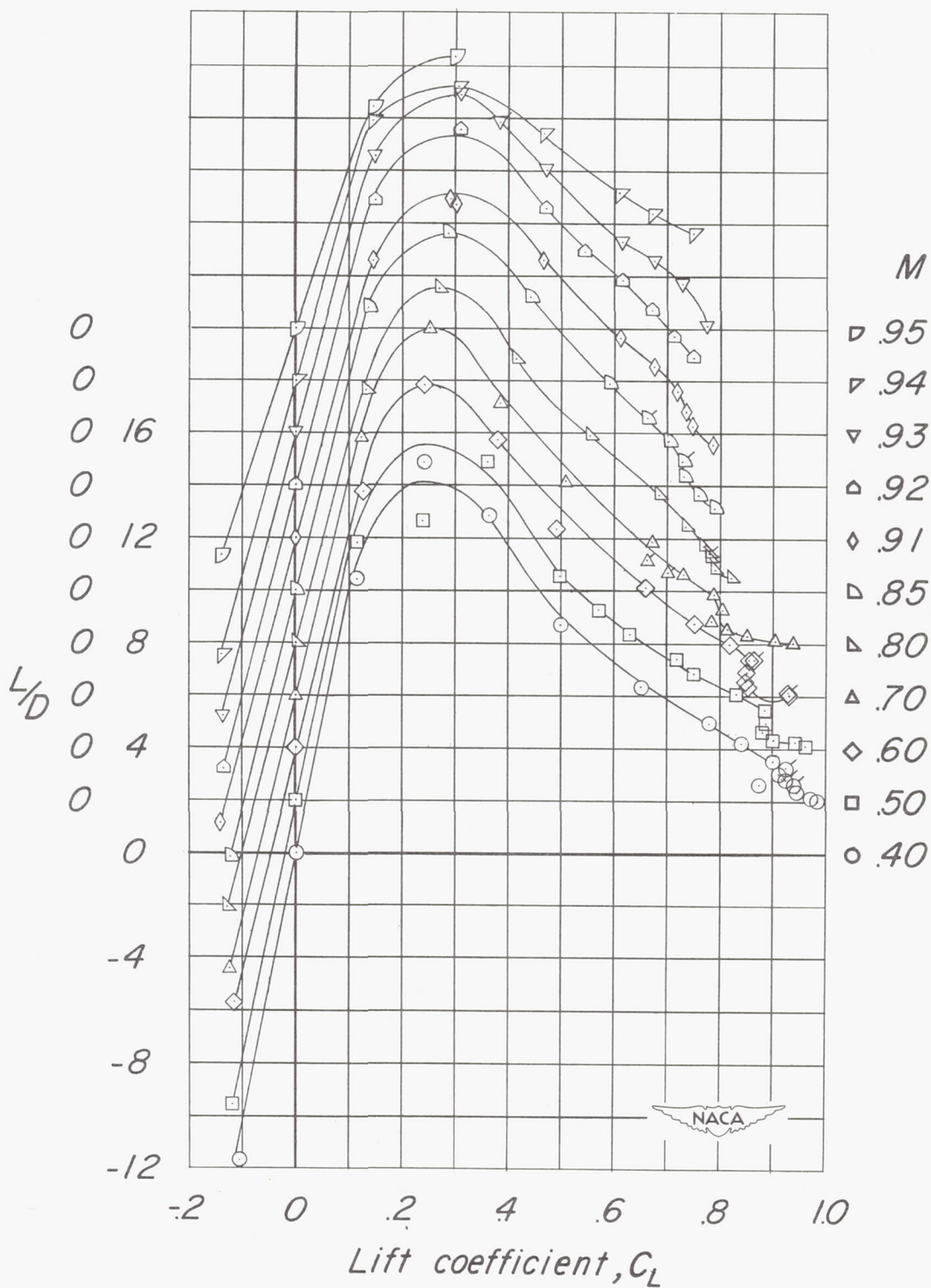
(d) Lift-drag ratios (45-4-1.0-006).
