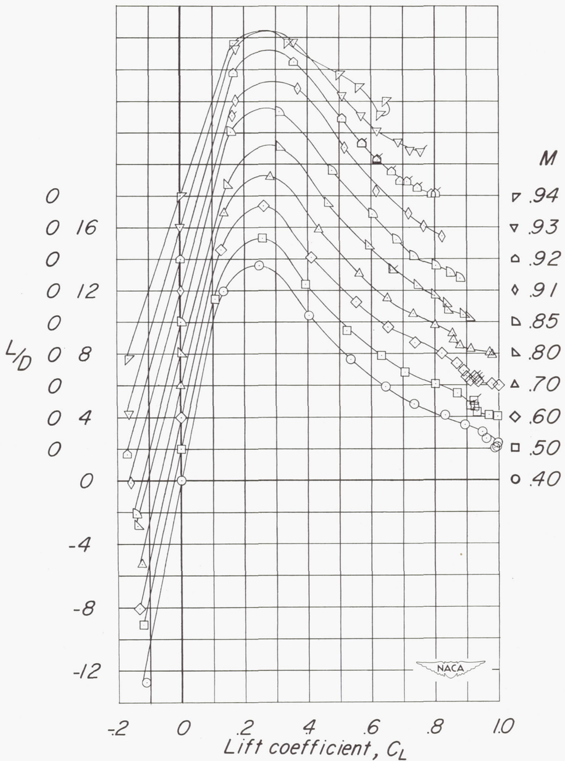
(d) Lift-drag ratios (45-4-0.3-006).
