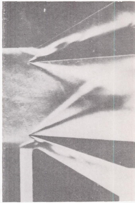
(d) Over-all total-pressure ratio, 7.22; plenum pressure, 1.19.
