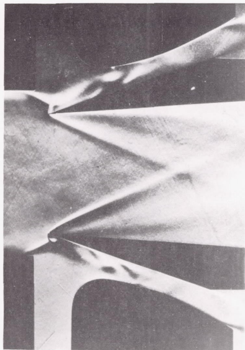
(d) Contraction ratio, 1.092; plenum pressure, 1.709.
