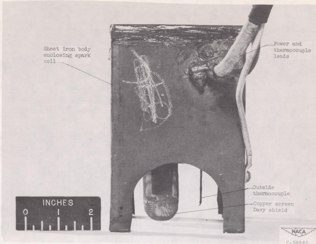
Figure 33. - Vapor Detector.
