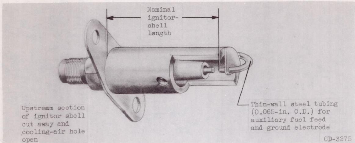
(d) Ignitor C.
