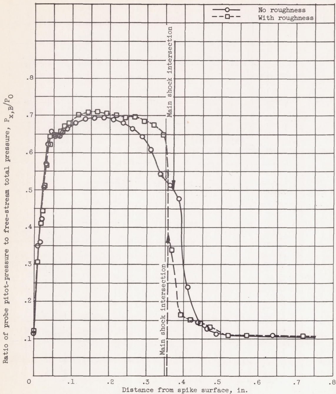
(d) Configurations D' and D'(R).
