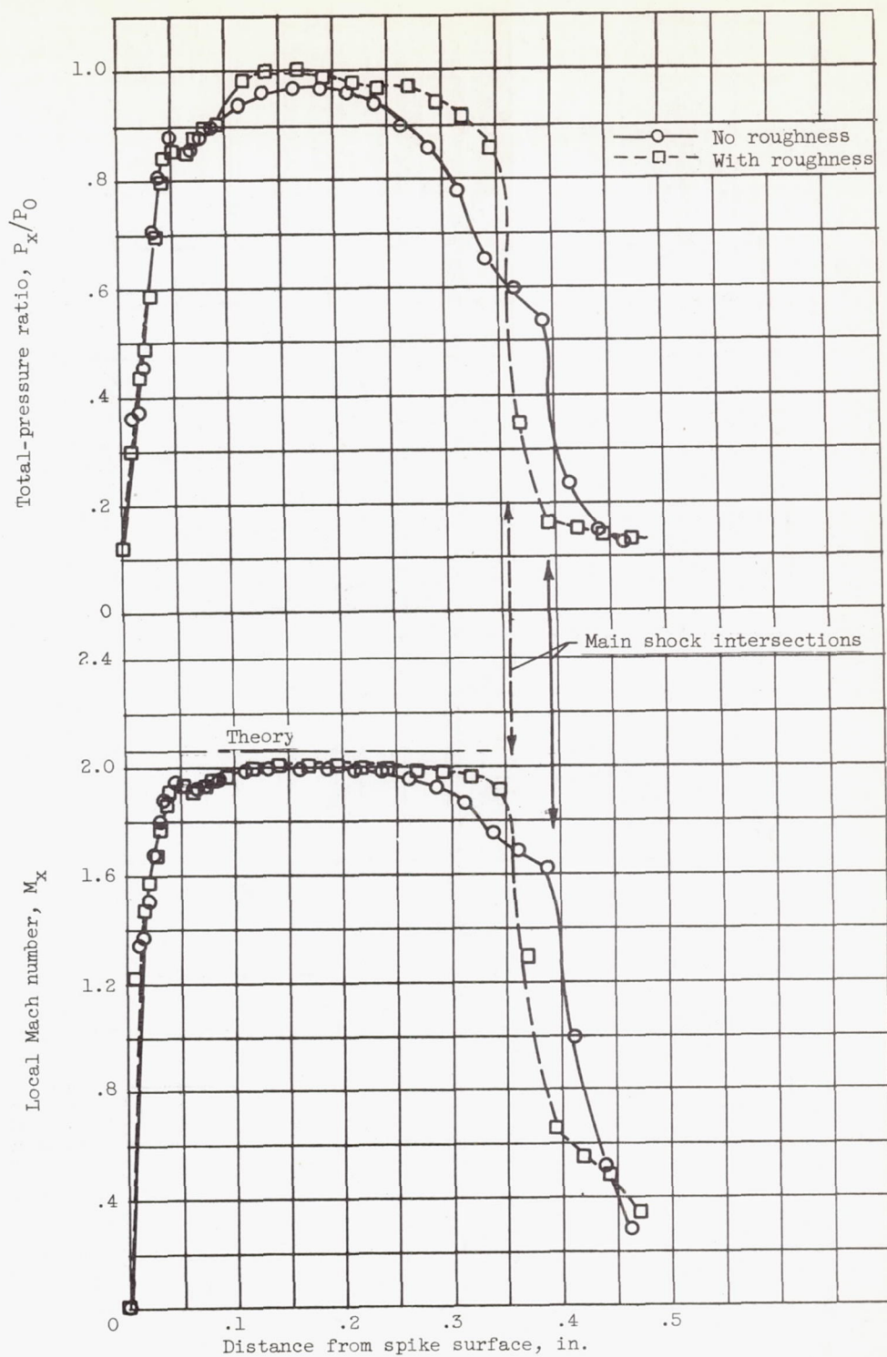
(d) Configurations D' and D'(R).
