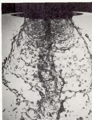
(d) Impinging-sheets injector; butt orientation of sprays.
