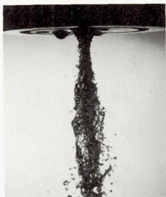
(d) Impinging-sheets injector; butt orientation of sprays.
