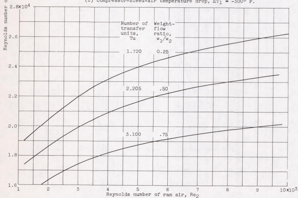
(d) Compressor-bleed-air temperature drop, \Delta T_1 = -400^\circ \text{F} .
