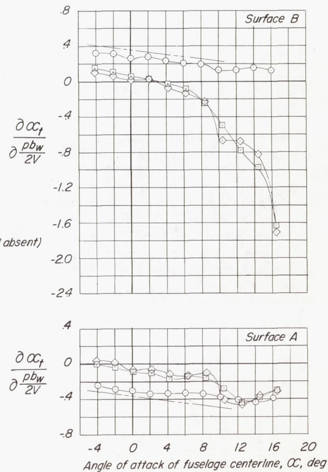
(d) Spanwise station, y = 6 inches.
