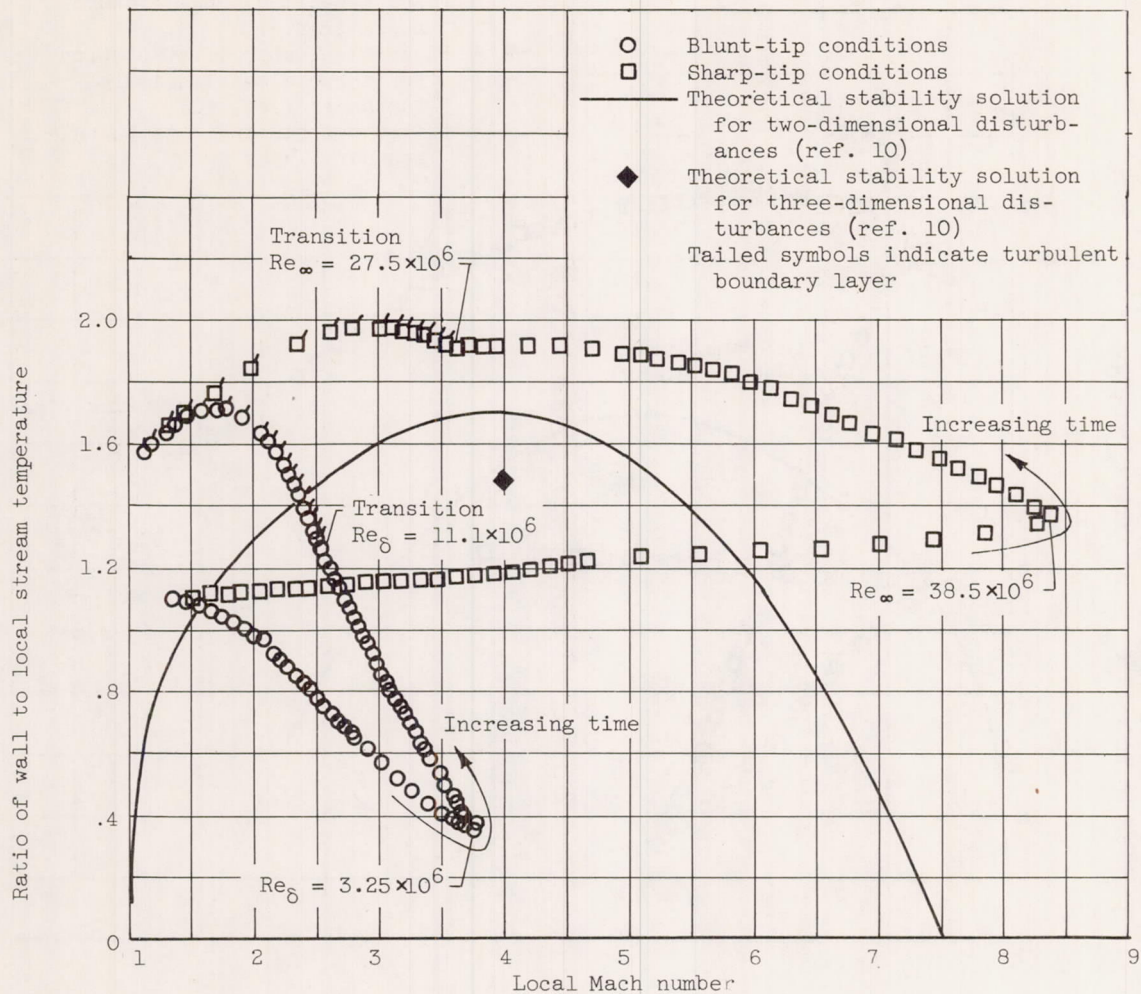
(d) Station 29.50.
