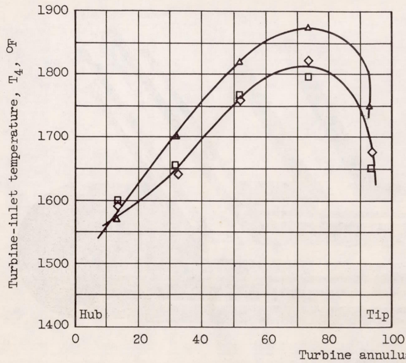
(a) Combustor A.
