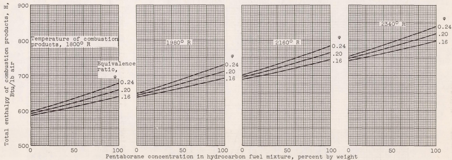
(d) Total enthalpy of combustion products.
