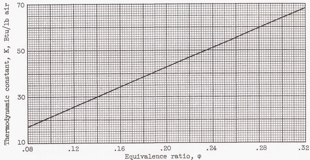
(d) Thermodynamic constant.
