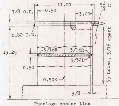
(d) Trailing-edge jet-spoiler details.
