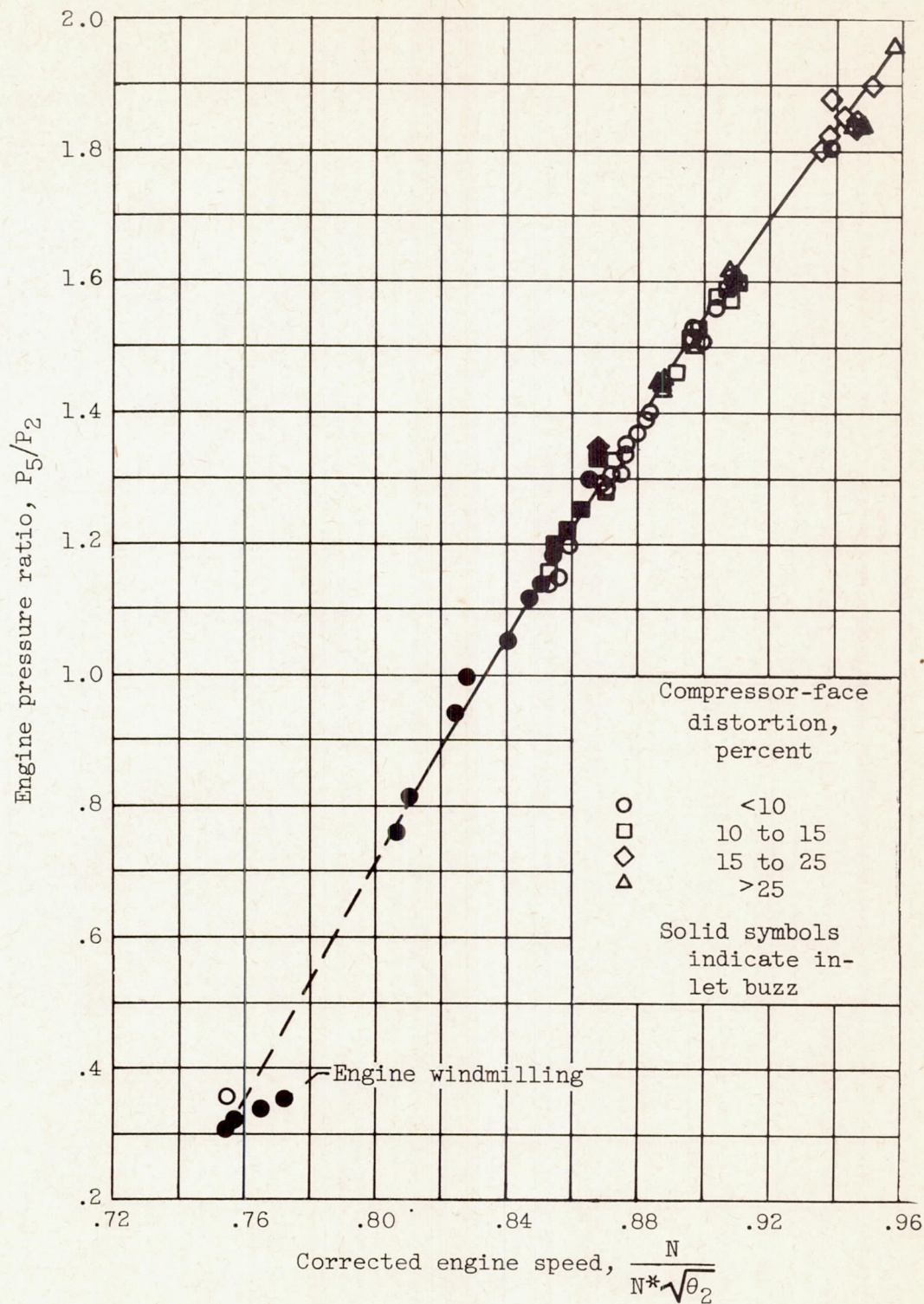
(d) Pressure ratio.
