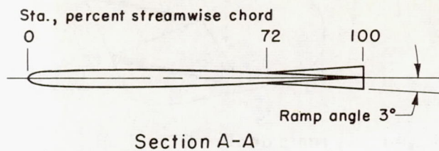
(d) Blunt trailing edge; ramp angle = 3^\circ .
