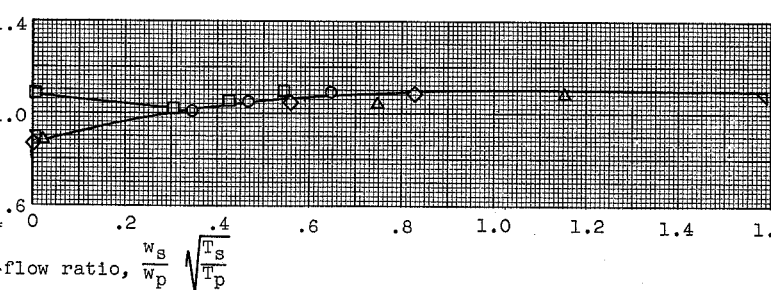
(d) No afterburning; Mach number, 1.0; d_s/d_p , 2.14.
