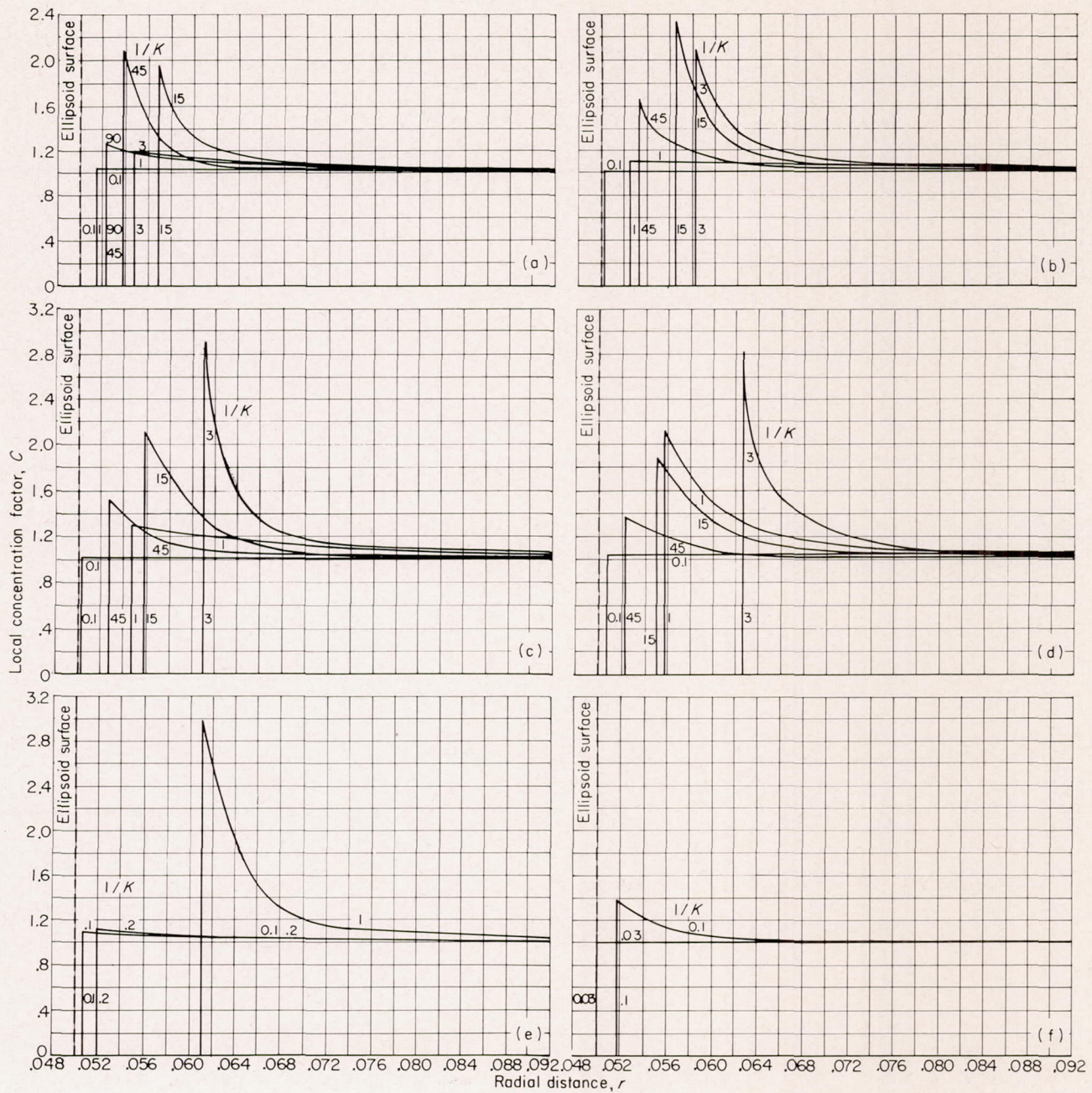
(a) z=0; Re_0=0 . (b) z=0; Re_0=128 . (c) z=0; Re_0=512 . (d) z=0; Re_0=1024 . (e) z=0; Re_0=4096 . (f) z=0; Re_0=8192 .
