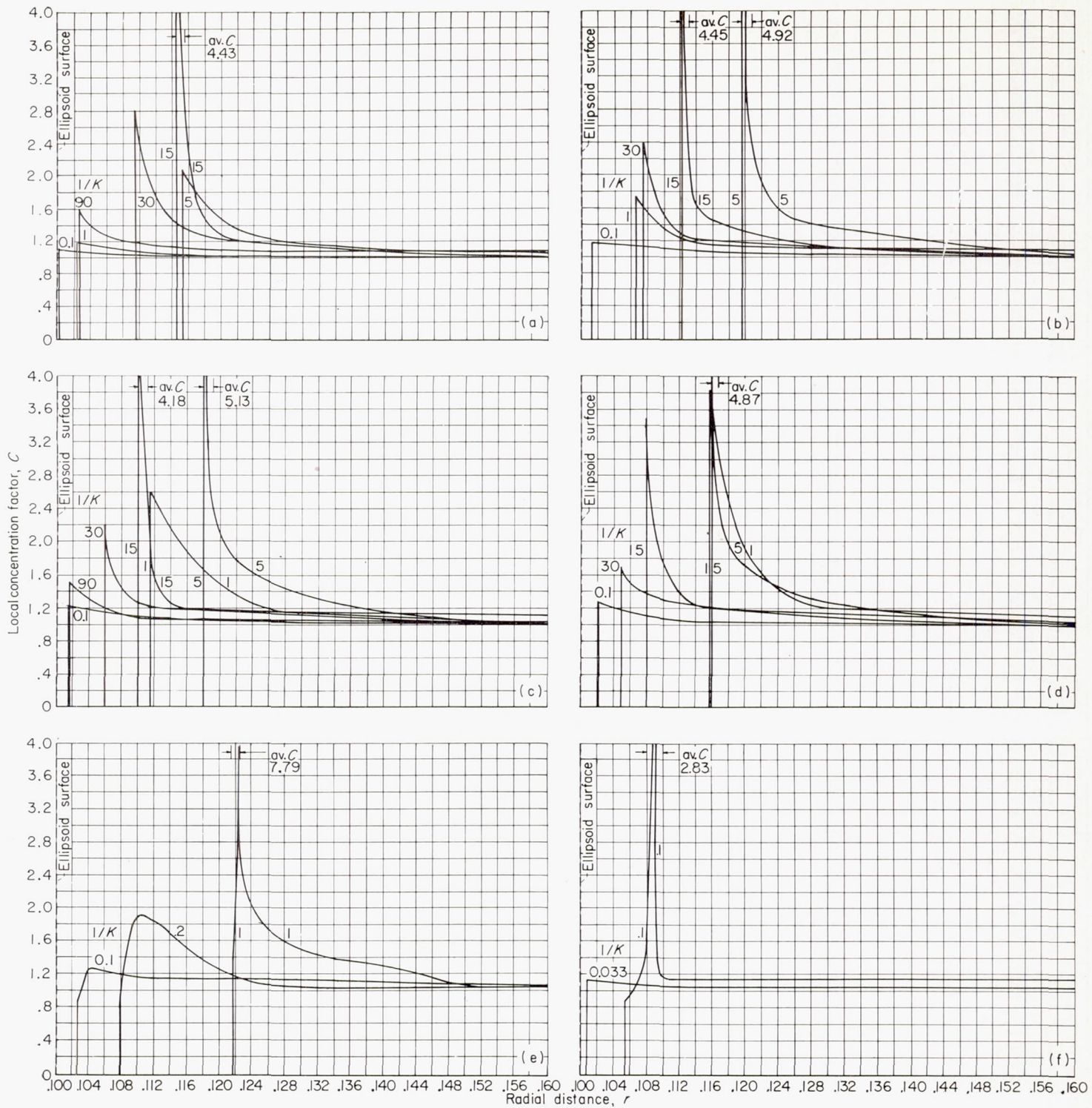
(a) z=0; Re_0=0 . (c) z=0; Re_0=512 . (e) z=0; Re_0=4096 .
