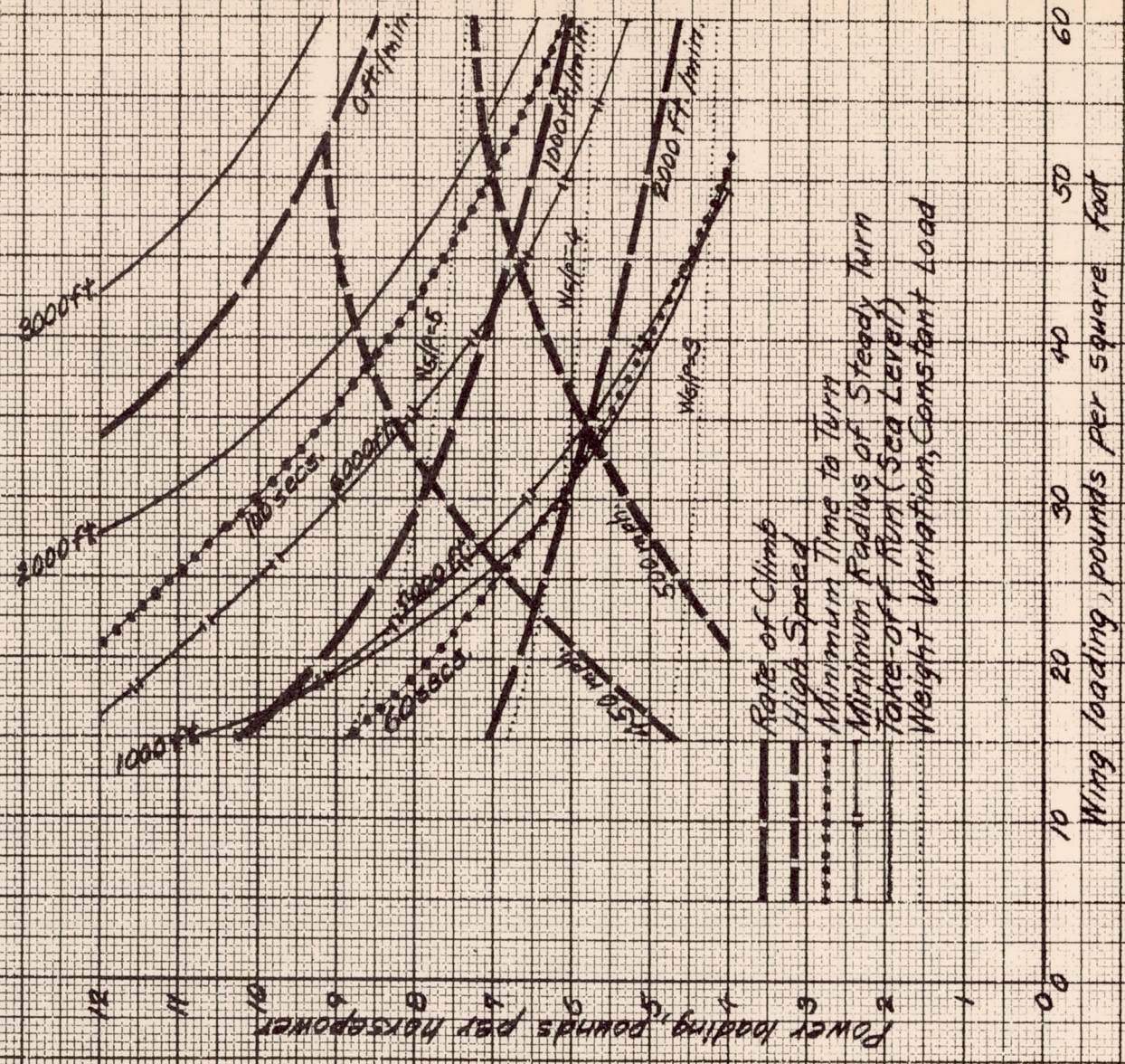
FIGURE 1 (d) - COMPOSITE SELECTION CHART - 40,000 FEET ALTITUDE R = 5.75
