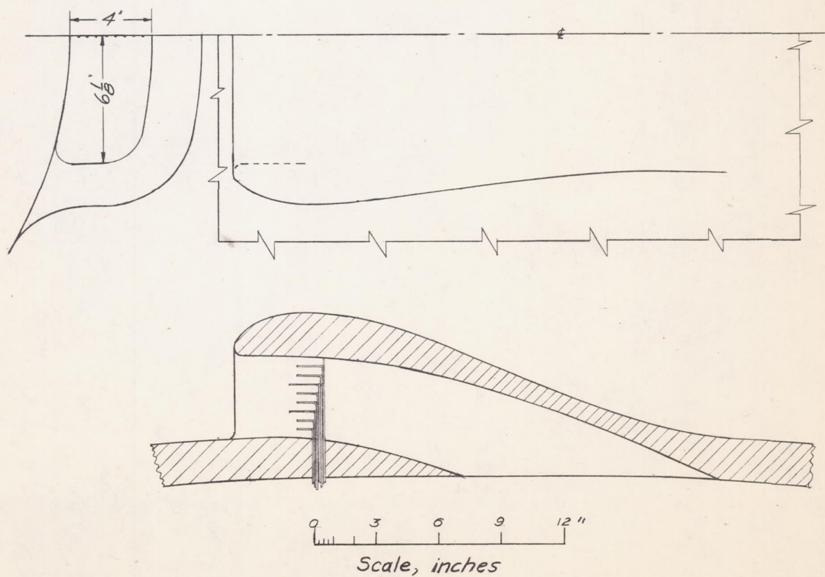
Figure 5.- Scoop B-1.
