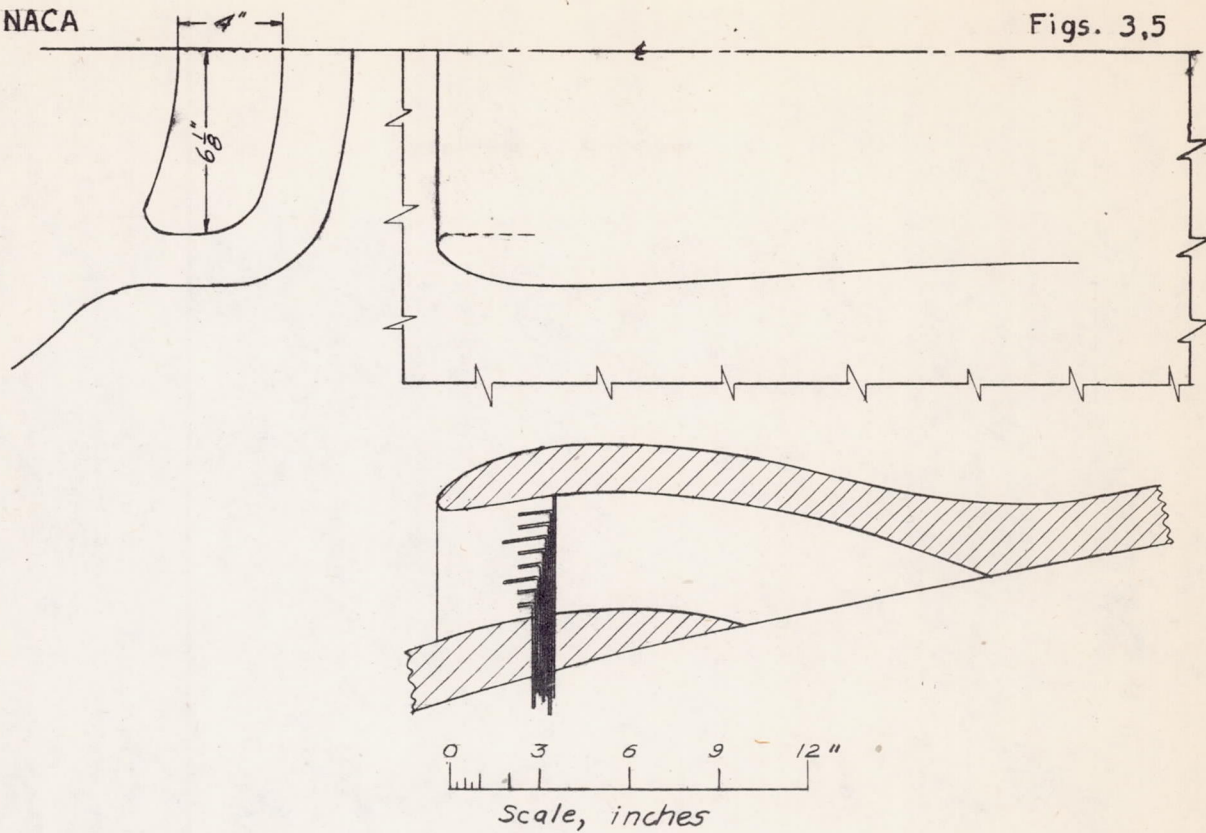
Figure 3.- Scoop A-1.
