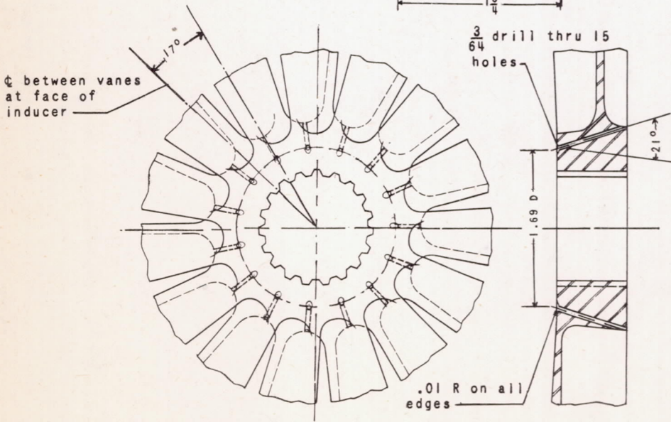
(d) Drilled inducer.
