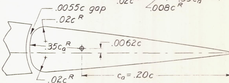
(d) Blunt-nose-balance aileron on the NACA 23012 airfoil.
