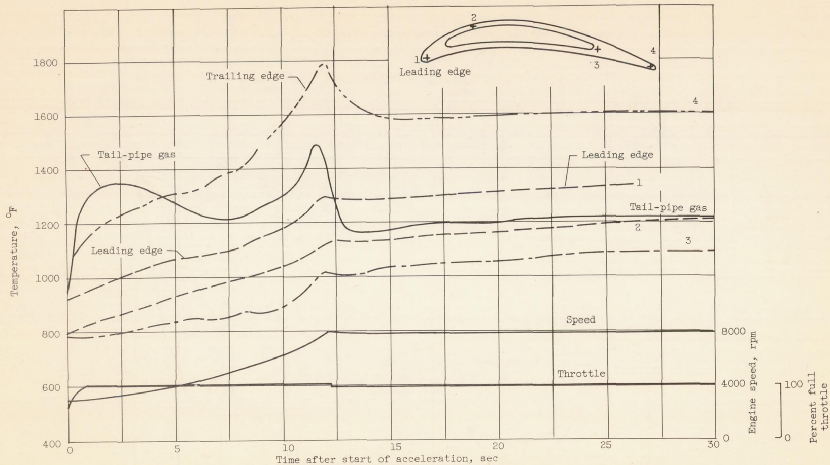
(b) Nozzle guide vane.
