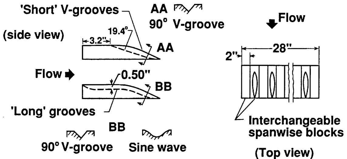
(d) Longitudinal grooves.
