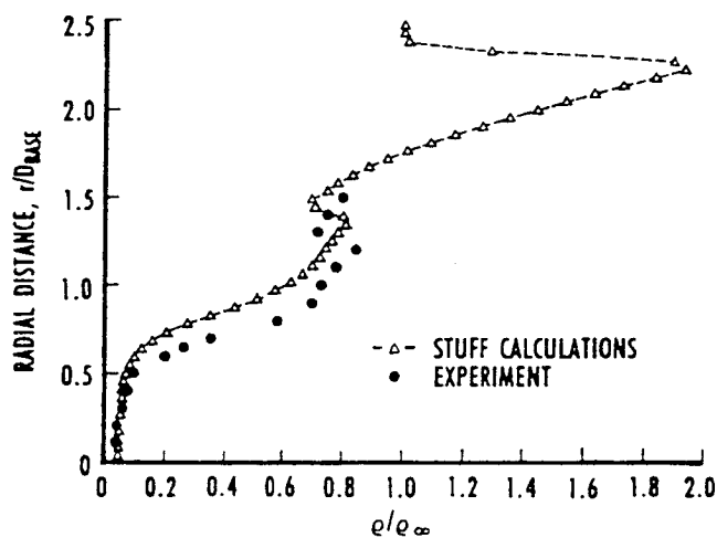
a. Density
