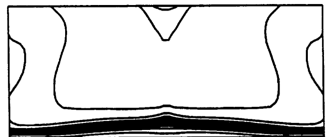
c) Mach 16
