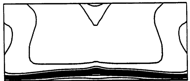
b) Mach 14
