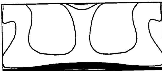
a) Mach 12
