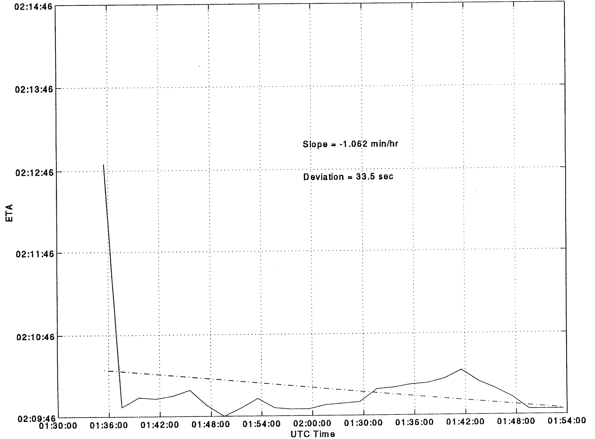
ETA vs Time for coa1765
