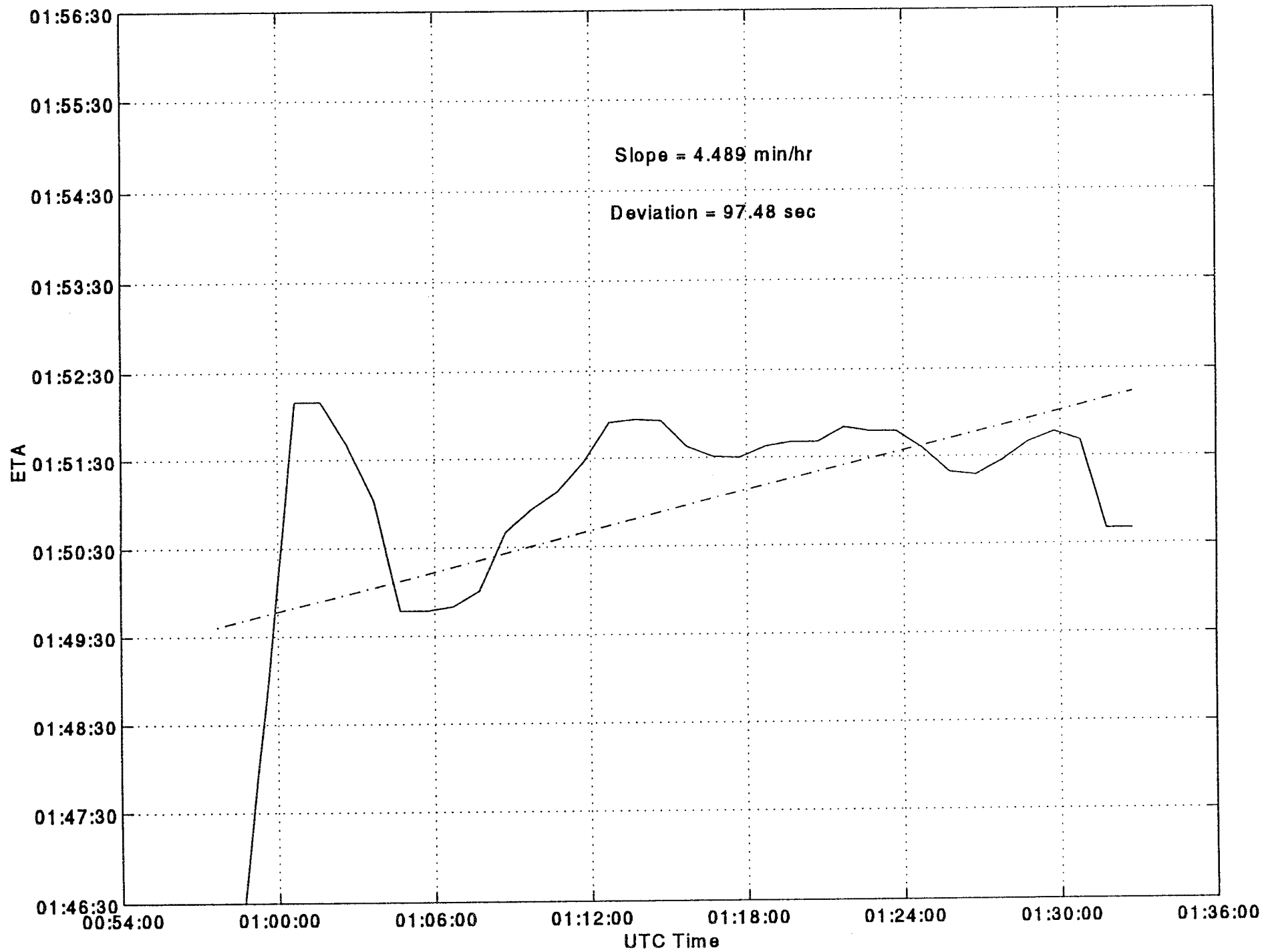
ETA vs Time for bta2296
