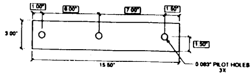
PL1 (5 REQD)
