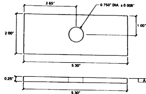
M4 (1 REQD)
