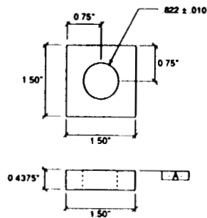
M2 (1 REQD)
