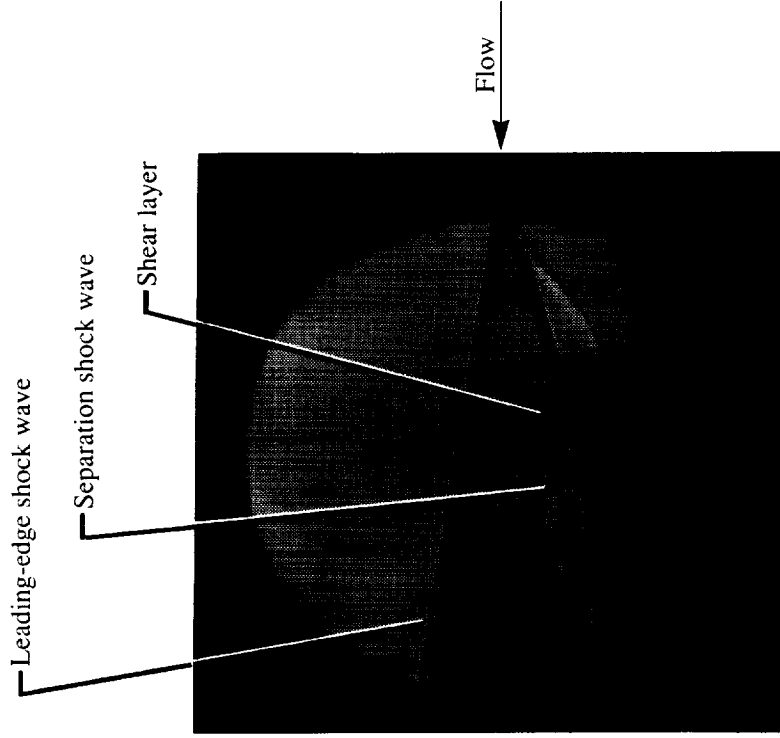
(b) Schlieren.
