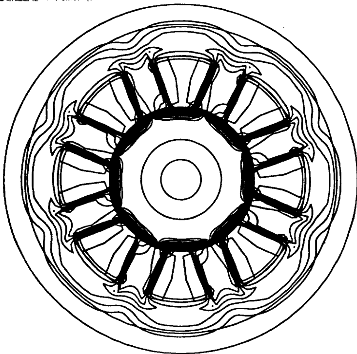
c) 995 rpm
