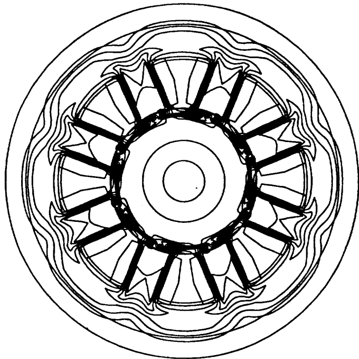
b) 95.5 rpm
