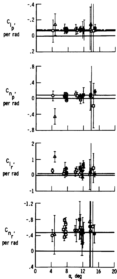
(d) C_{l_p} , C_{n_p} , C_{l_r} , C_{n_r} .
