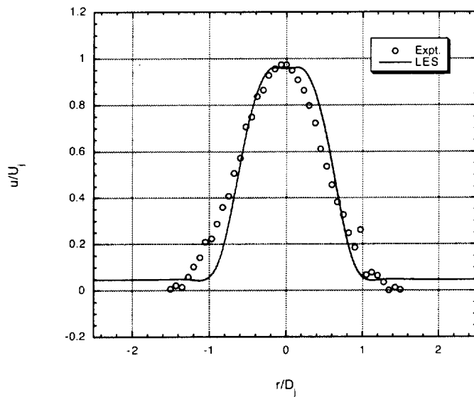
(d) x/D_j = 8
