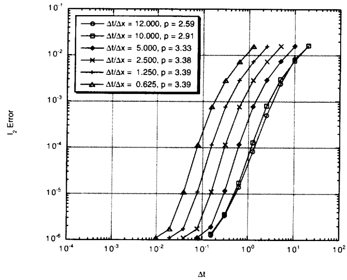
(b) Temporal error
