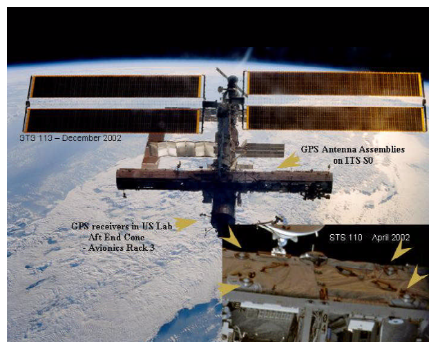
Fig. 2 ISS GPS subsystem.
