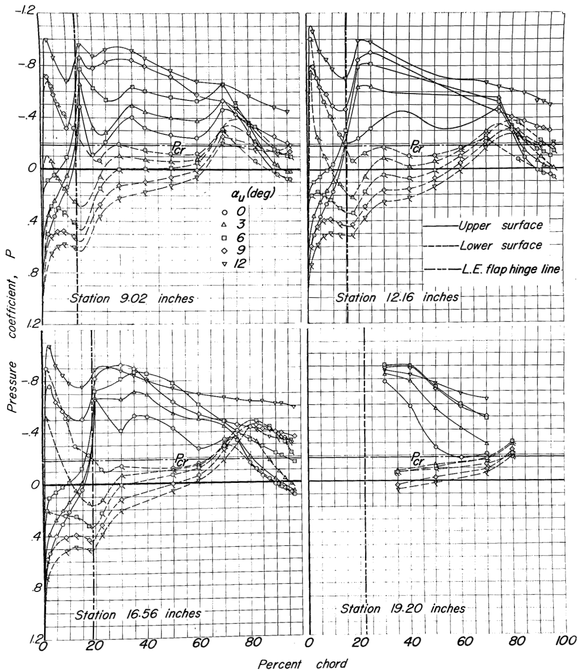
(d) Mach number, 0.90.
