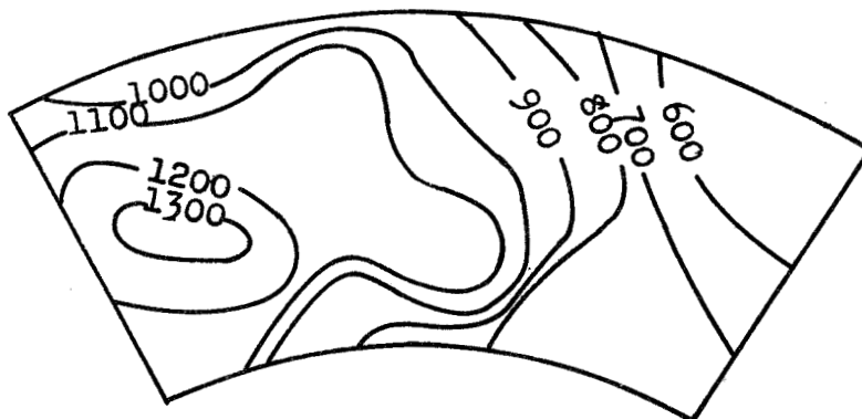
(d) Modification 3. Average combustor-outlet temperature, 953° F.
