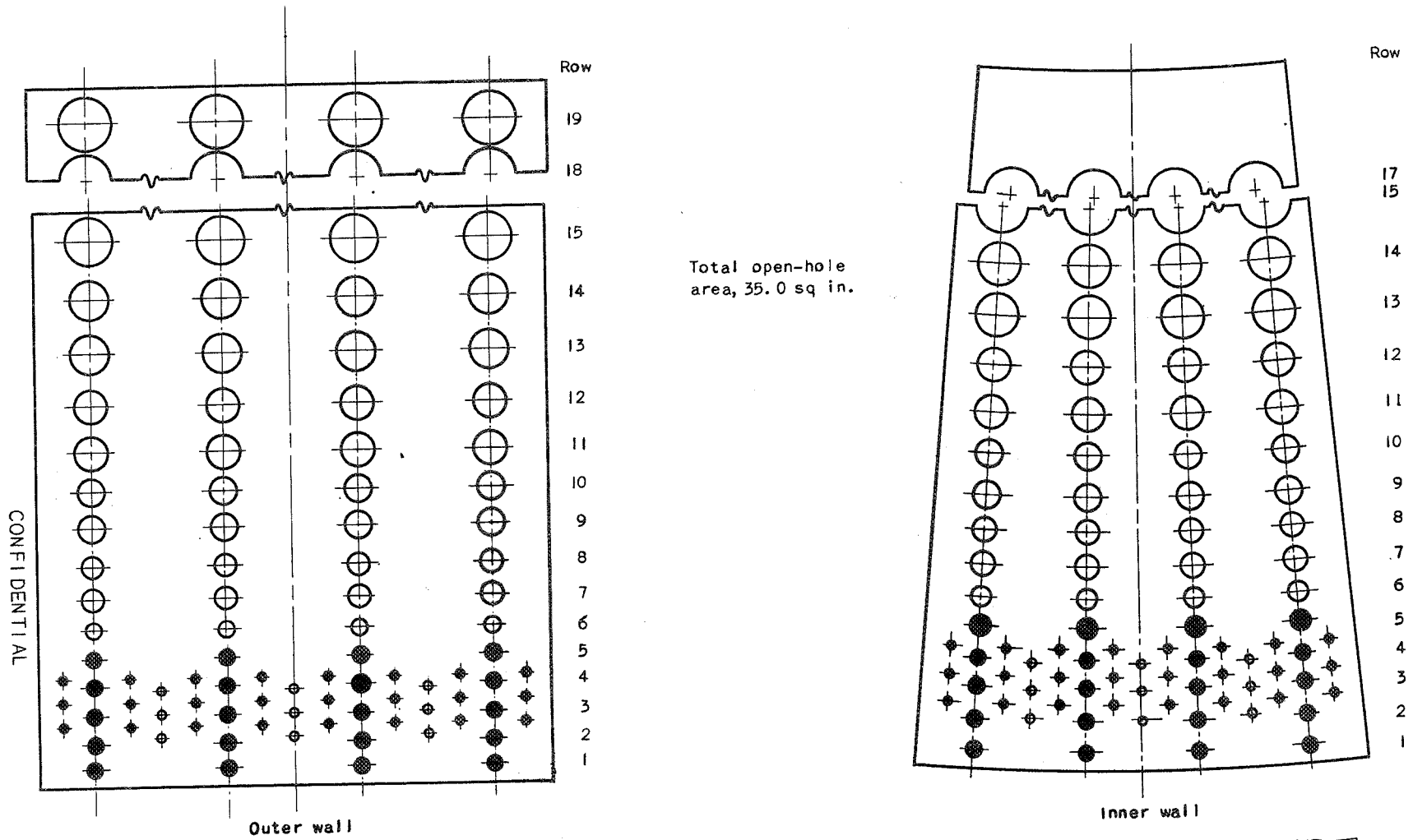
(d) Modification 3 (shaded holes blocked).
