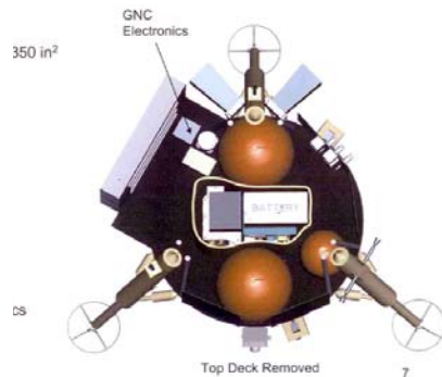
VEB Enclosure
