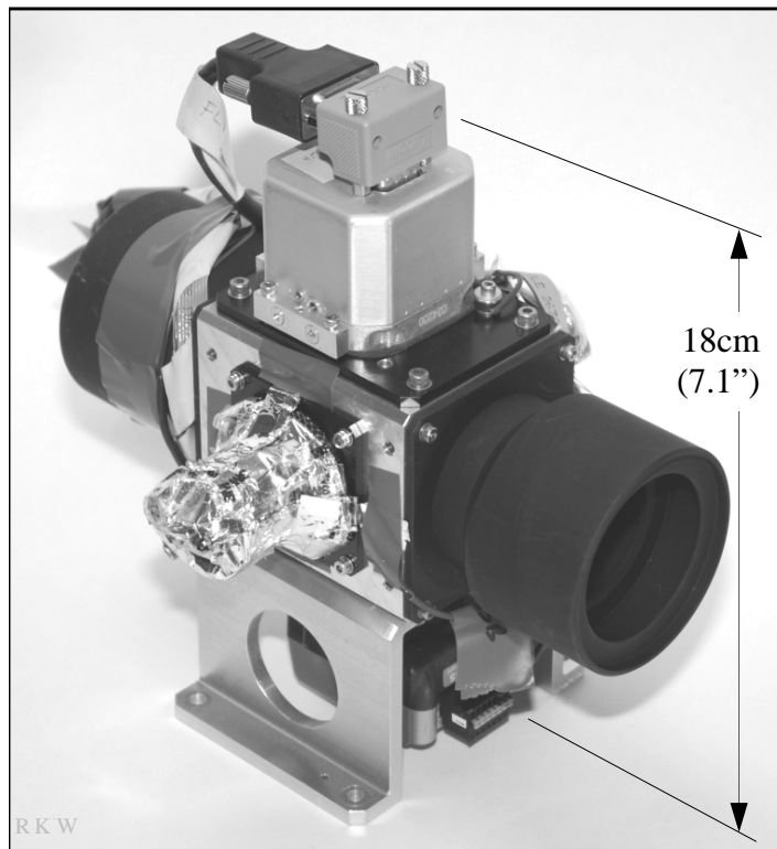
Figure 1. BESST Radiometer
