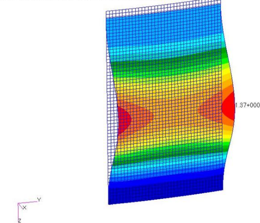
Panel B-2 (Average I.D. Bow)
