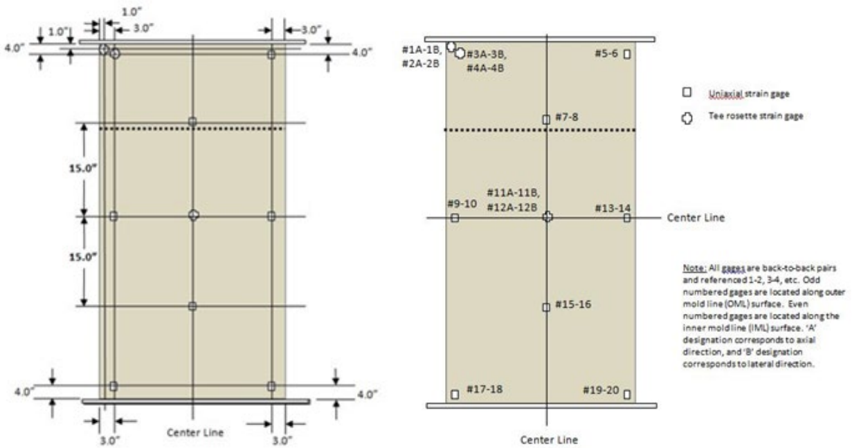
a.) Panel B-1
