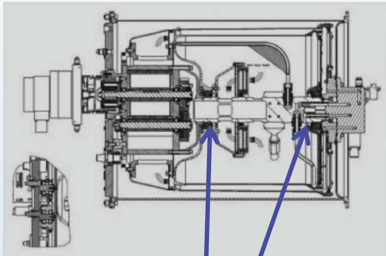
DA Cross Section
