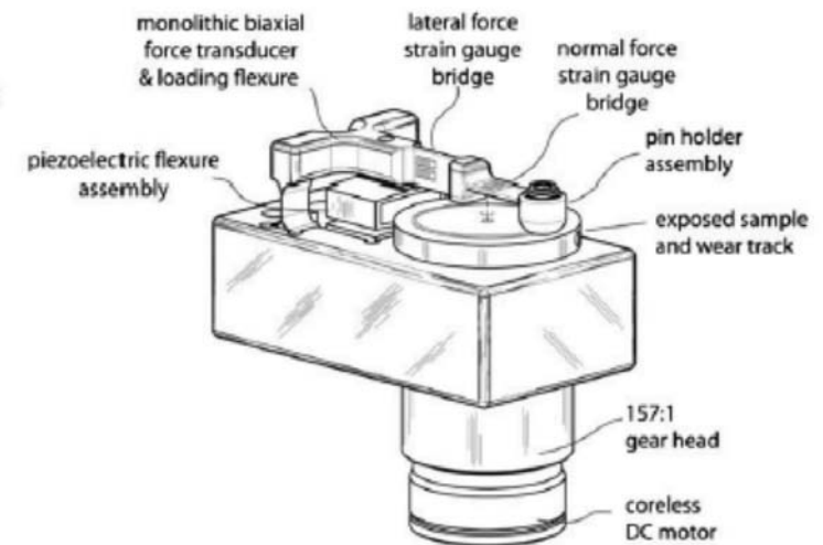
Pin-on-disk tribometer unit
