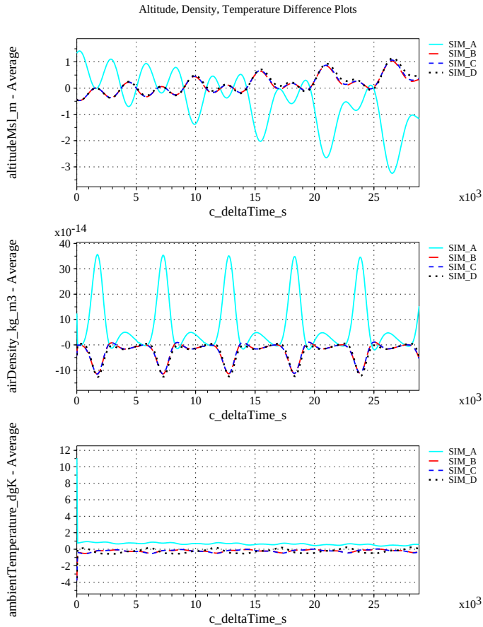
(d) Atmospheric Properties Differenced
