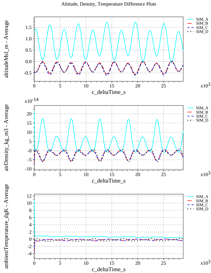
(d) Atmospheric Properties Differenced
