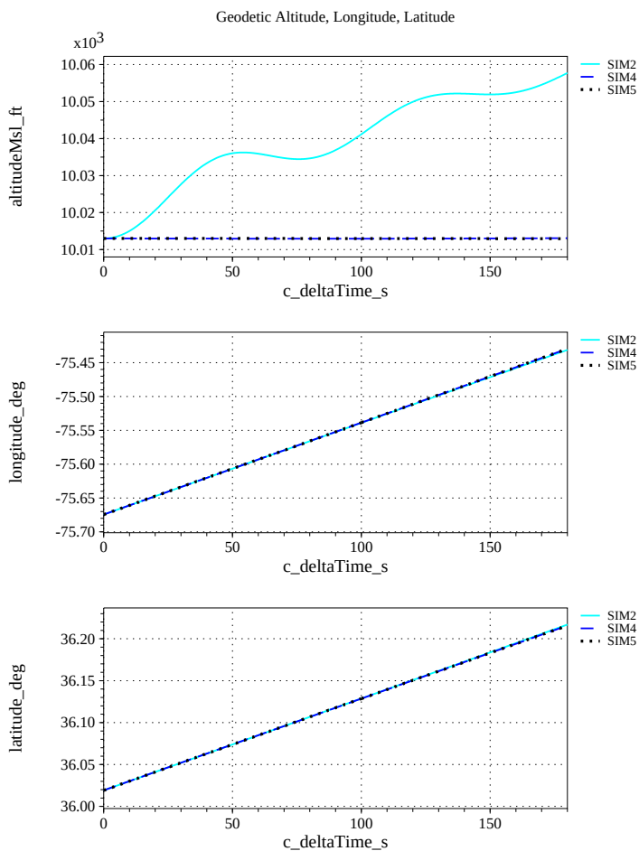
(e) Altitude, Geodetic Latitude and Longitude Compared
