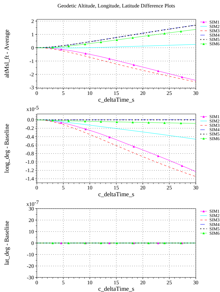
(f) Altitude, Geodetic Latitude and Longitude Differenced
