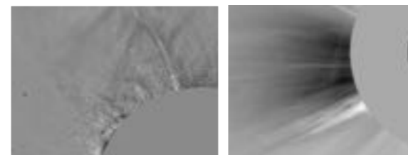
Hinode / XRT
