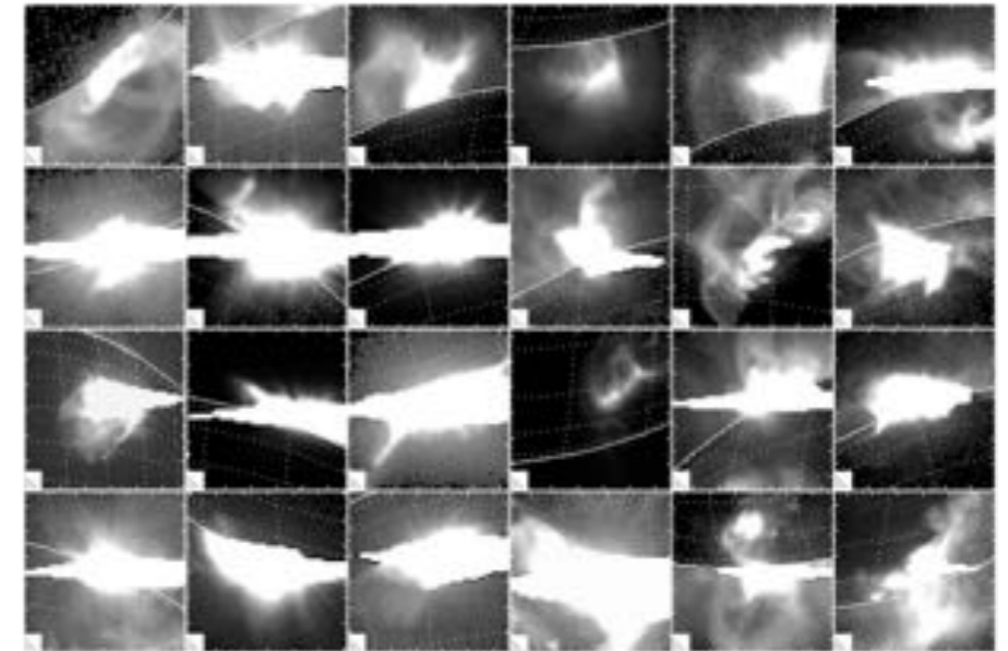
Yohkoh / SXT
