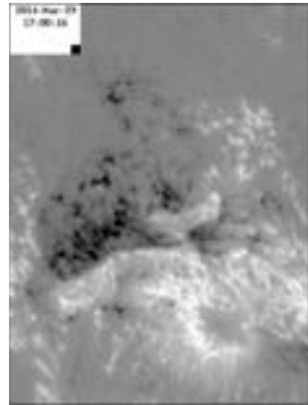
Hinode / XRT
