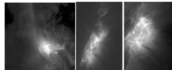
SOHO / LASCO
