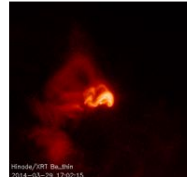
Hinode / XRT
