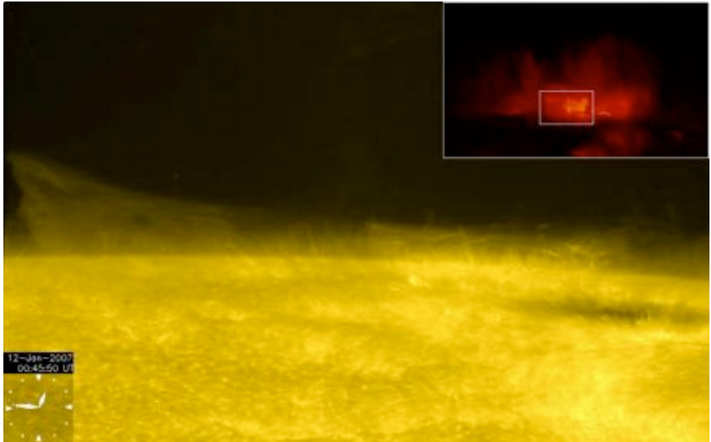
Hinode / SOT
