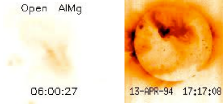
Yohkoh / SXT
