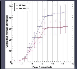
Fig 4: Cum. histogram of flash mag
