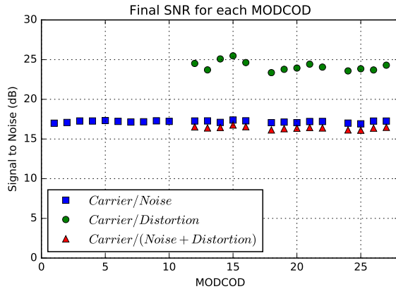
Fig. 12. SNR Metrics
