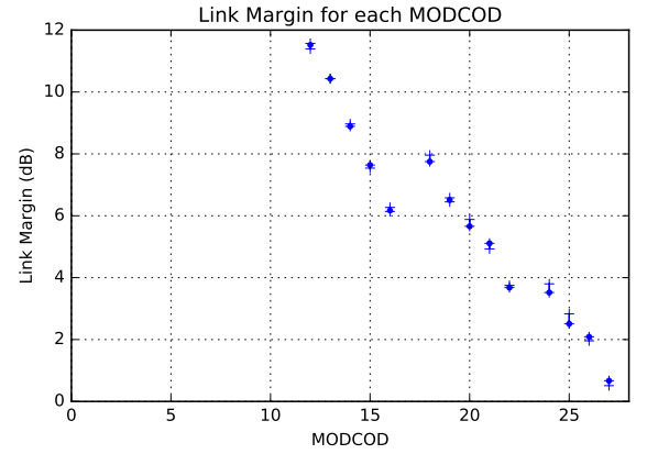
Fig. 11. Link Margin
