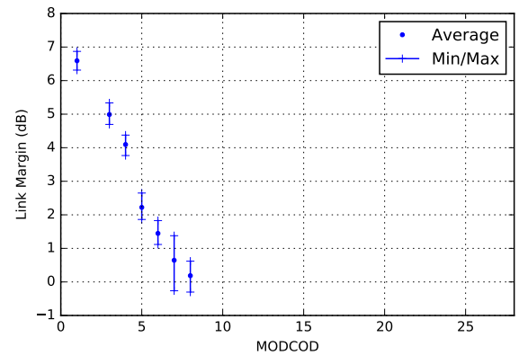
Fig. 23. Link Margin vs MODCOD
