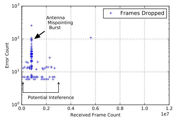
Fig. 17. Frame Count
