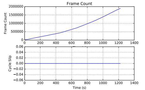
Fig. 13. Frame Count
