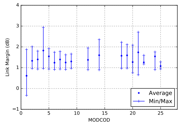
Fig. 15. Link Margin vs MODCOD
